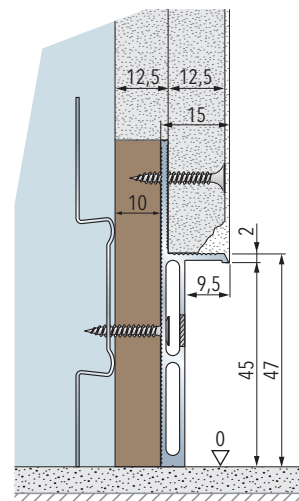
Soklový profil na SDK stene s dvojitým opláštením
