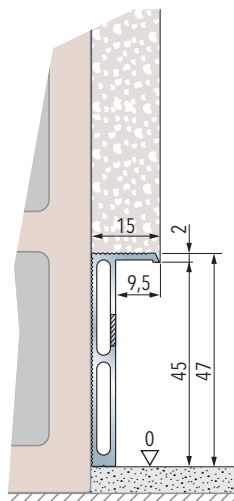
Soklový profil na murovanej stene
