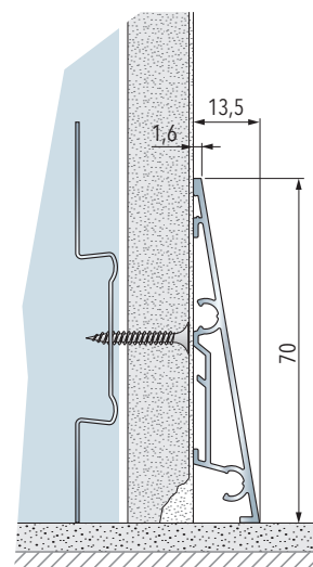
Soklová lišta inštalovaná na sadrokartónovej stene (jednoduché opláštenie).
