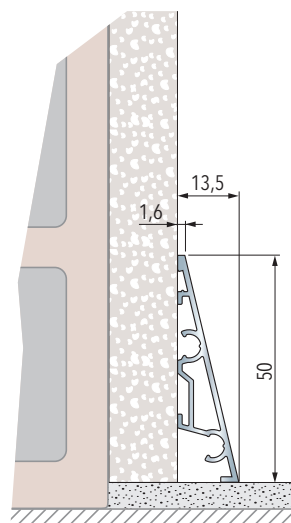
Soklová lišta inštalovaná na murovanej stene.
